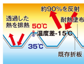
遮熱塗装の仕組み
